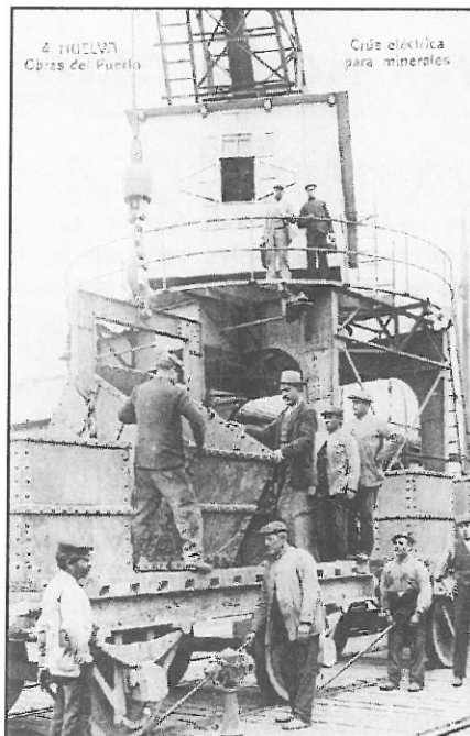
Grúa eléctrica y vagones utilizados para el movimiento mineralero en los muelles. El aumento en la exportación del mineral hizo que se fueran abandonando paulatinamente las grúas de vapor.
